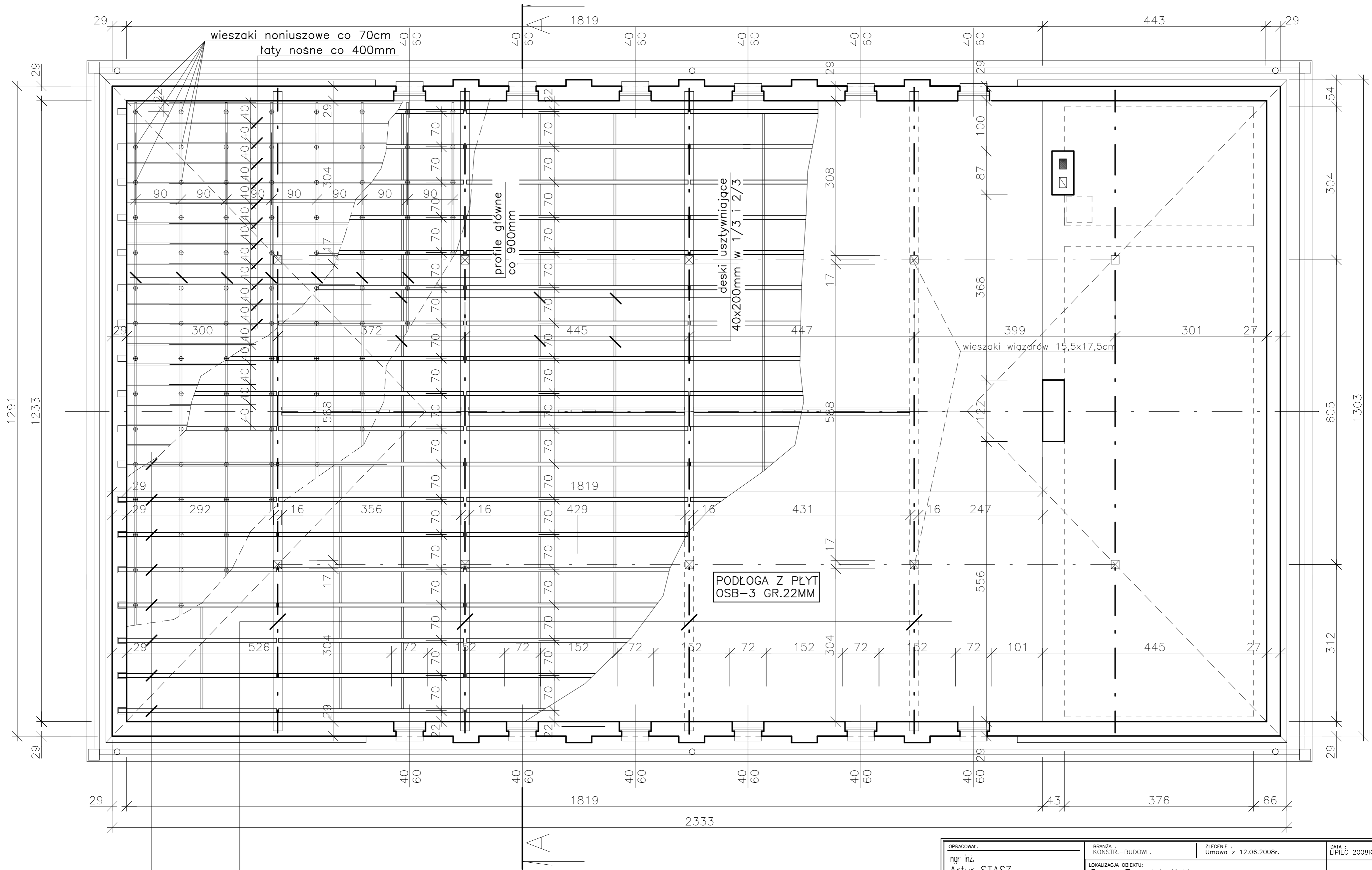
RZUT KONSTRUKCJI STROPU PODDASZA – 1:50
